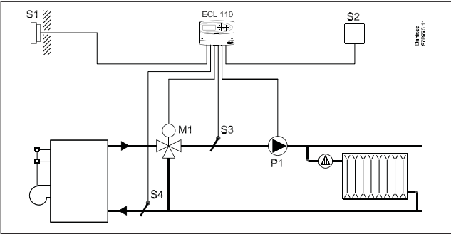
Värmesystem 2: Värmekrets med panna
